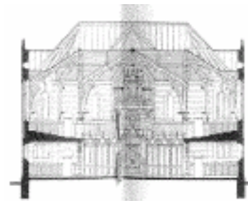
Querschnitt
