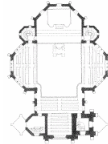
Emporen-Grundriss
