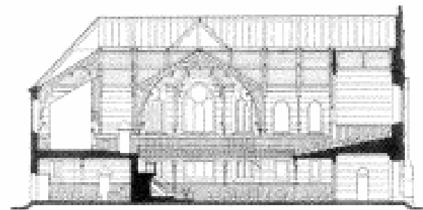
Längsschnitt
